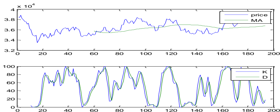
图 1 策略信号
