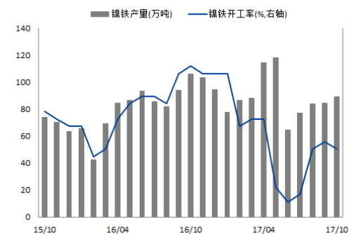
图 21 镍铁产量及开工率
