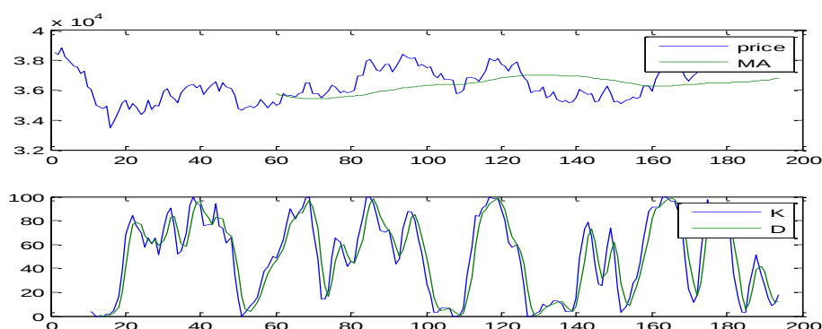
图 1 策略信号
